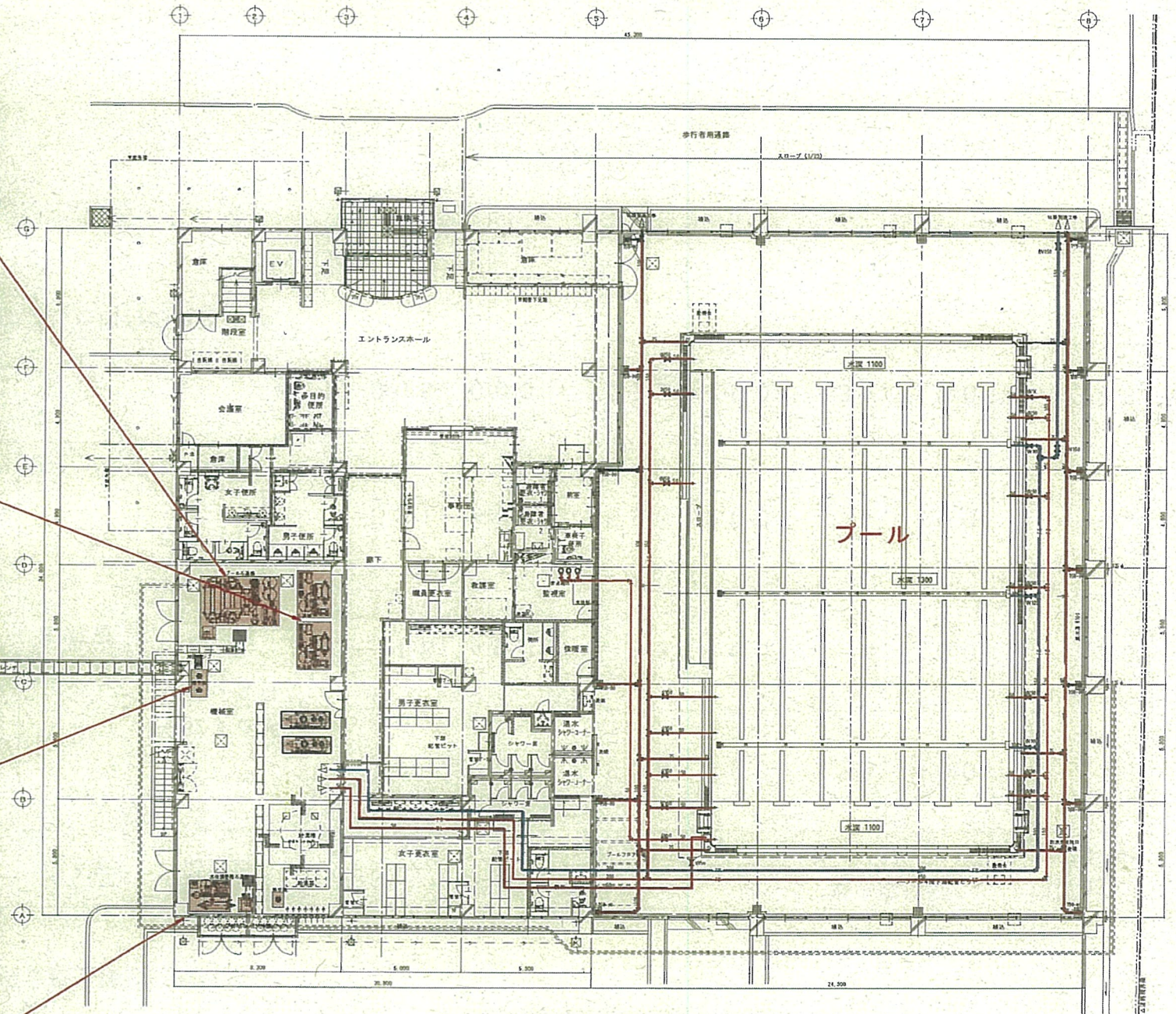
余熱利用施設 1階平面図
