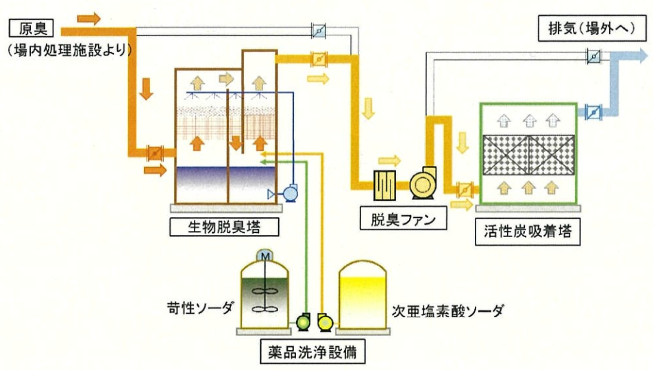
脱臭設備処理フロー(生物脱臭+活性炭)
