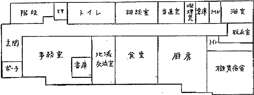
1階平面図
