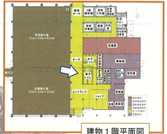
建物1階平面図
