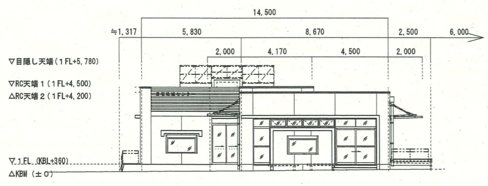
東側立面図
