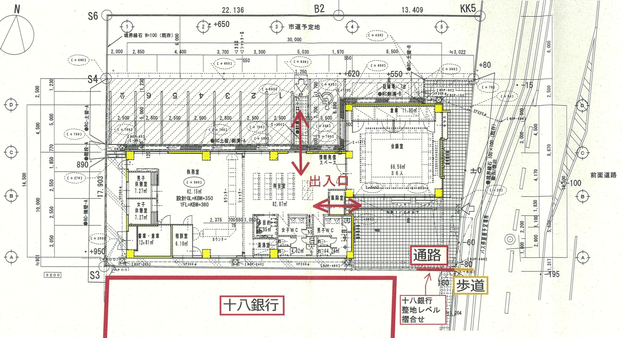
滑石地域センター配置兼平面図 S = 1 / 100
