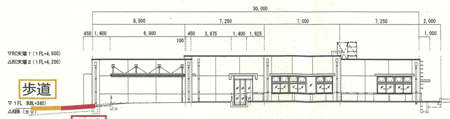
北側立面図
