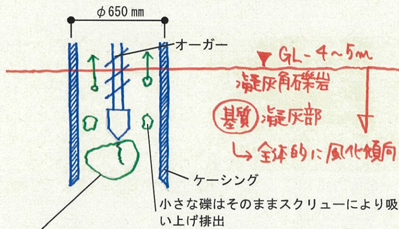
地中の掘削施工断面イメージ図(計画)
