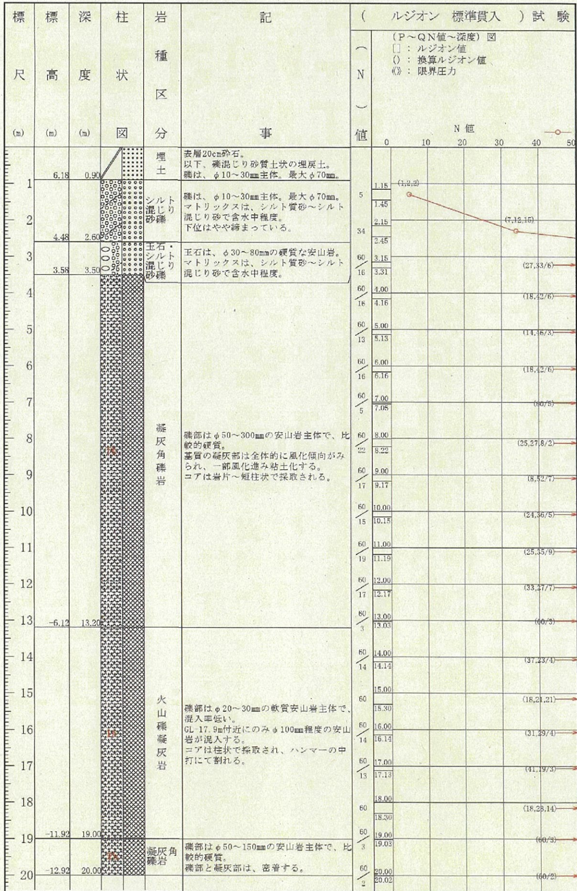
地質調査ボーリング NO.1 柱状図
