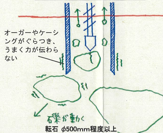
地中の掘削施工断面イメージ図(実施)
