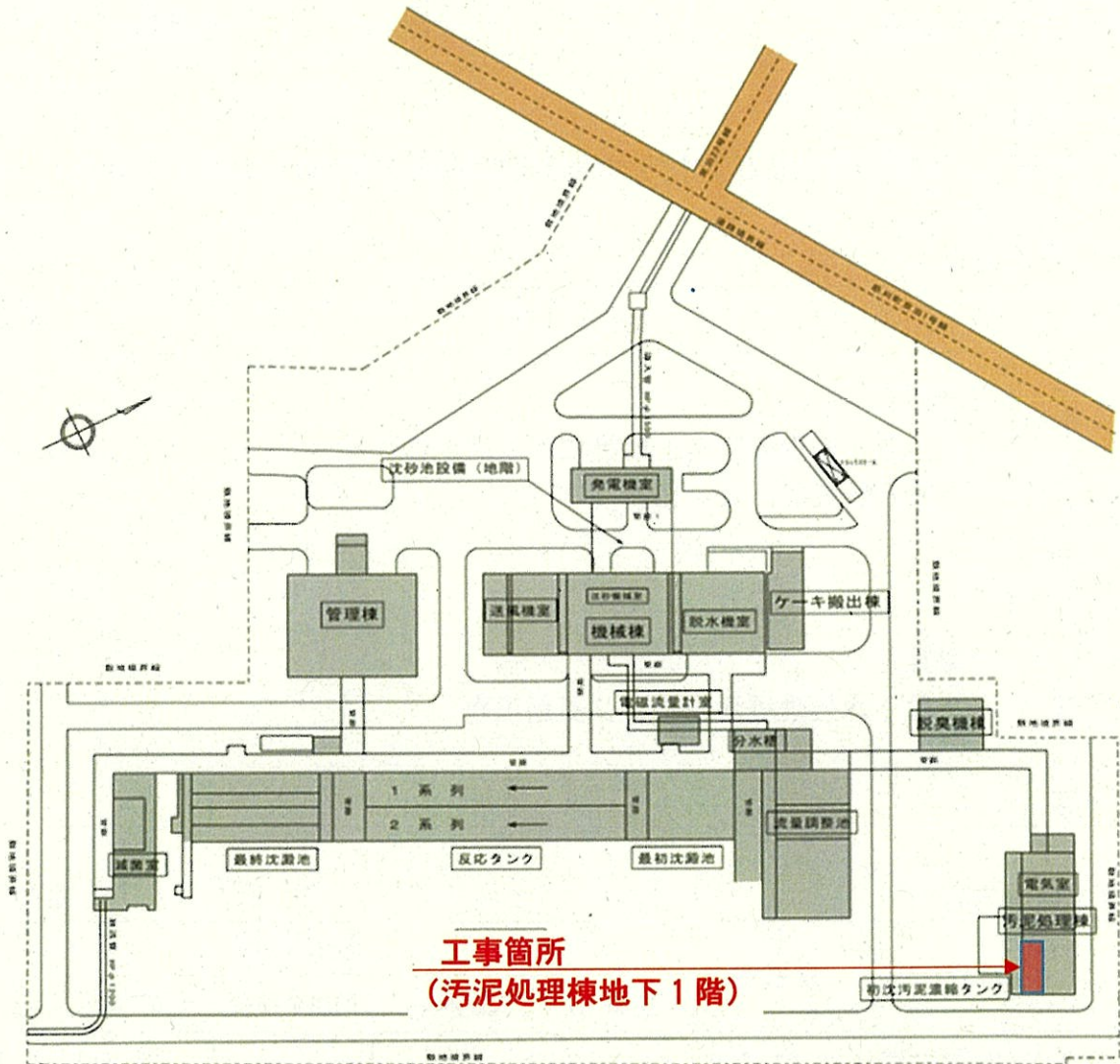
三重下水処理場平面図
