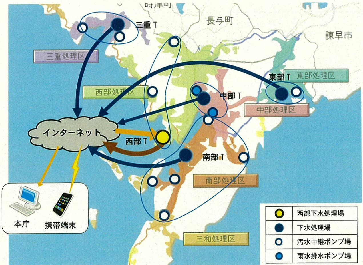
下水処理場・ポンプ場配置図
