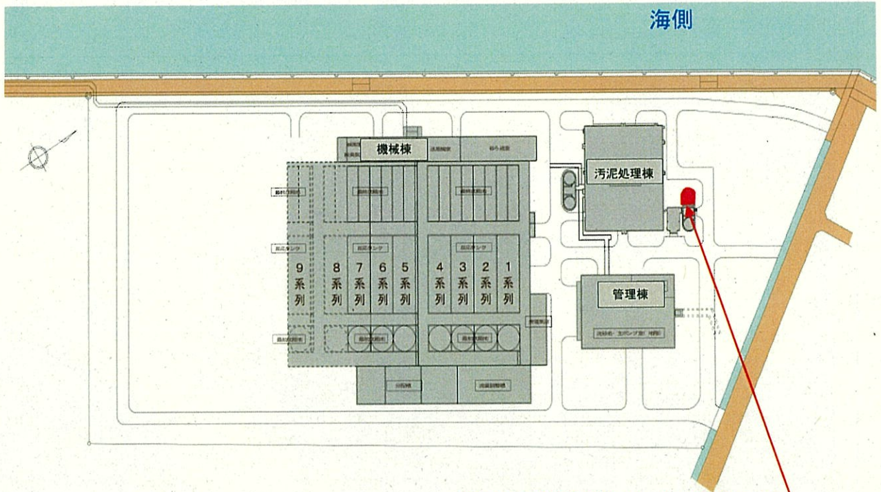
初沈汚泥濃縮槽（土木）築造工事
