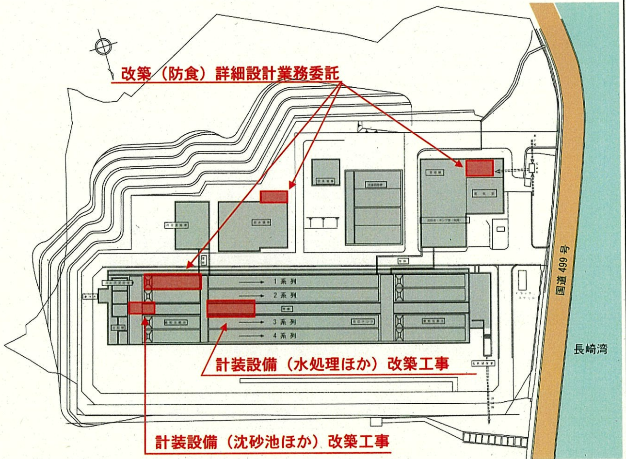
南部下水処理場平面図
