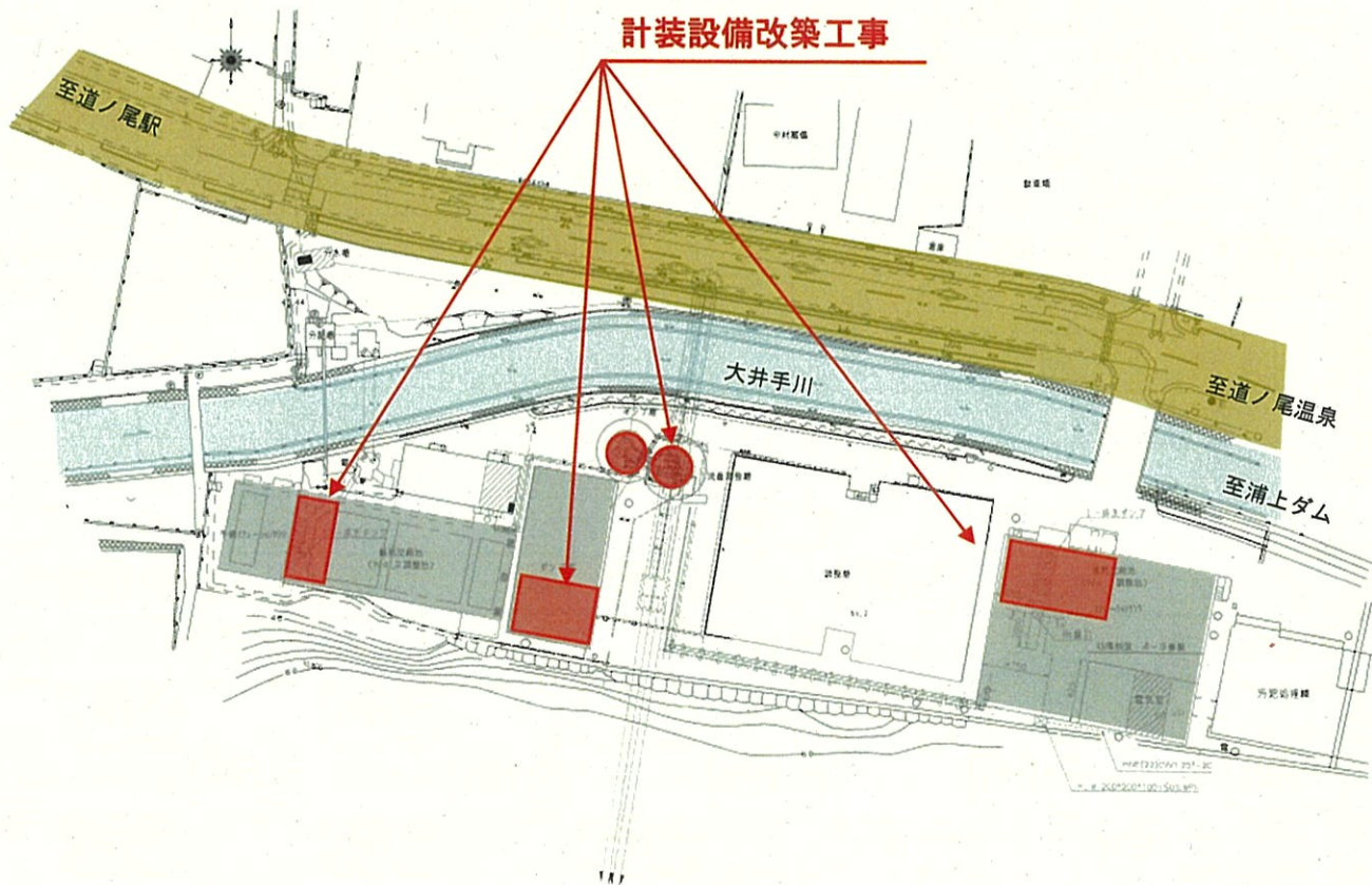
西部道ノ尾流量調整池平面図
