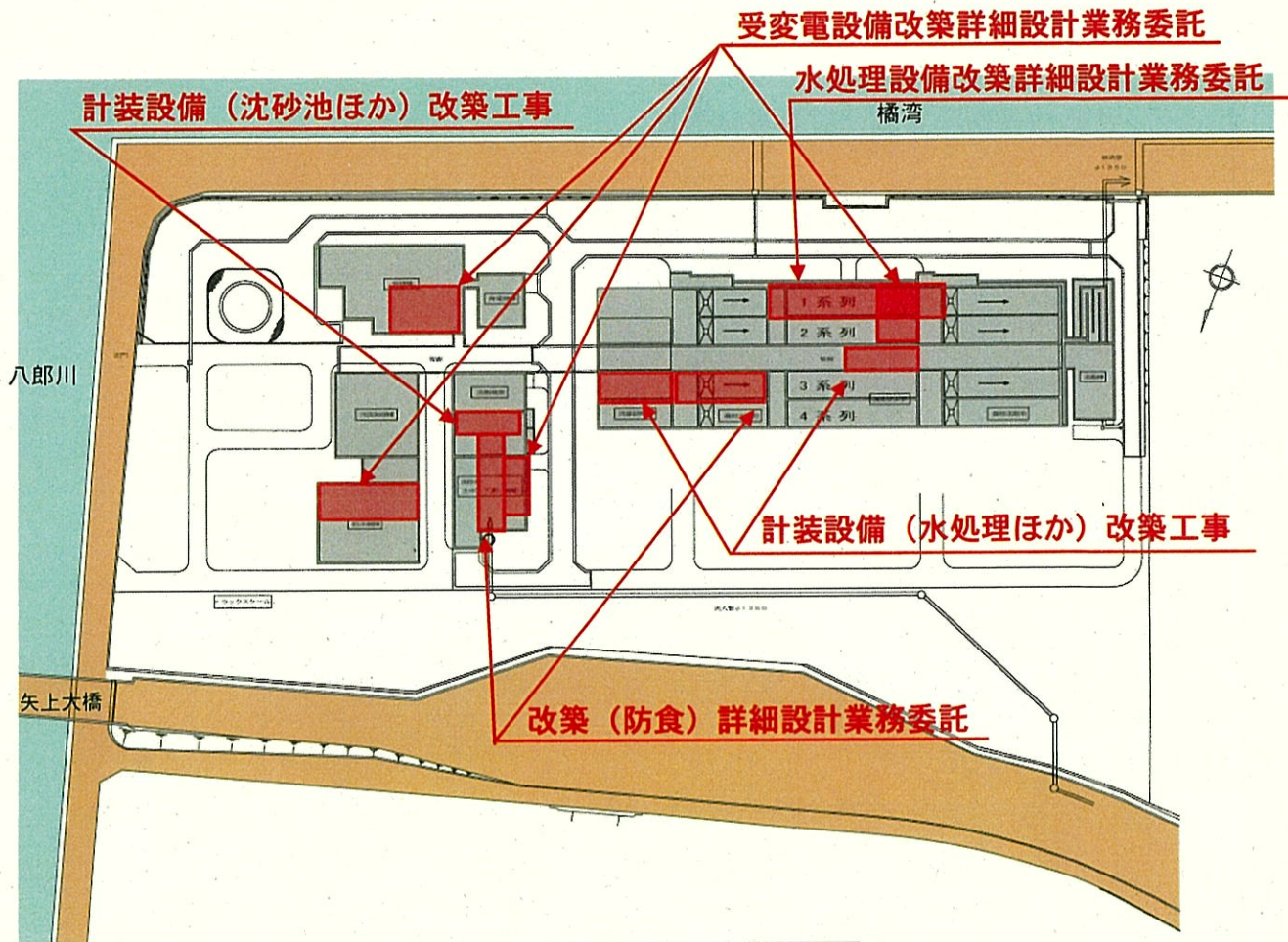
東部下水処理場平面図
