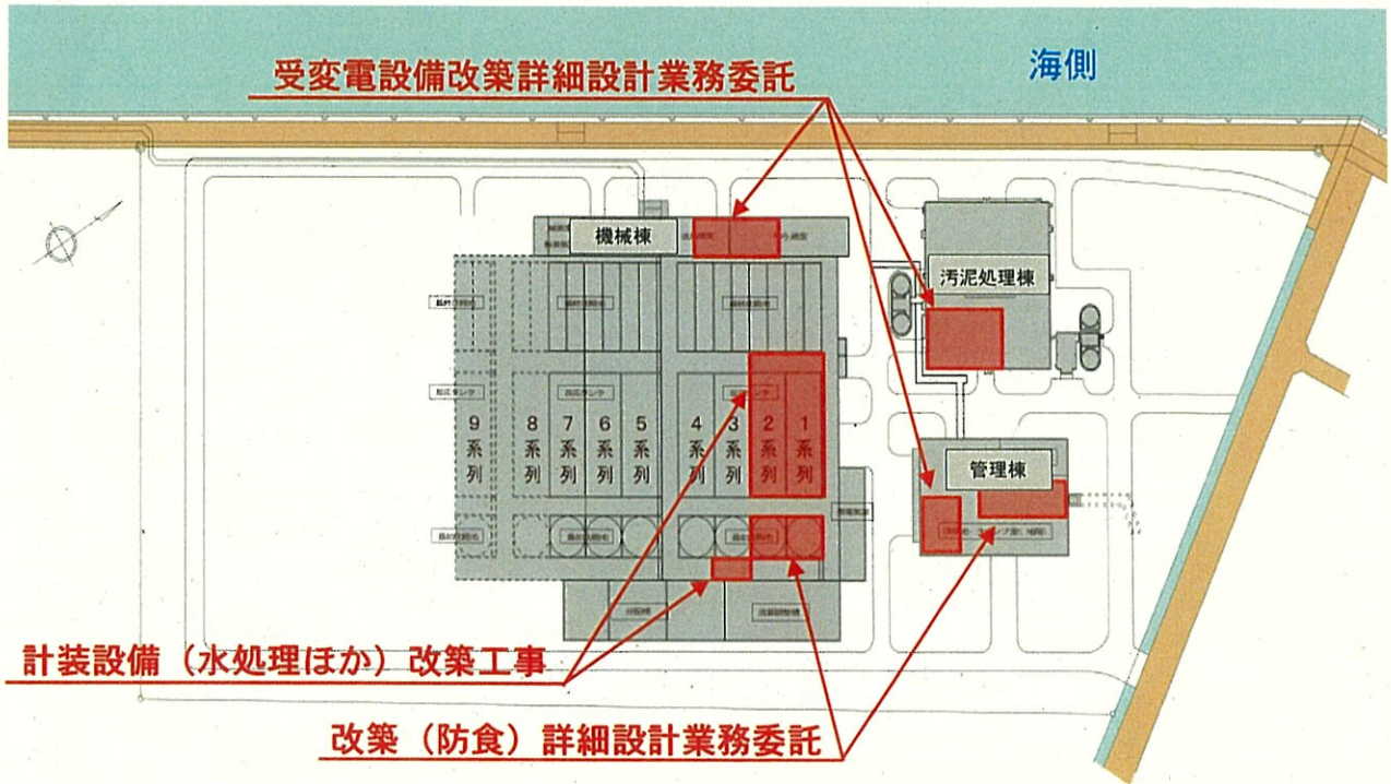
西部下水処理場平面図
