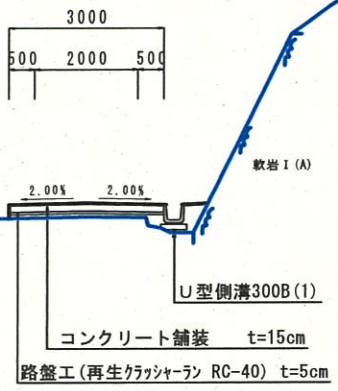
標準断面図
