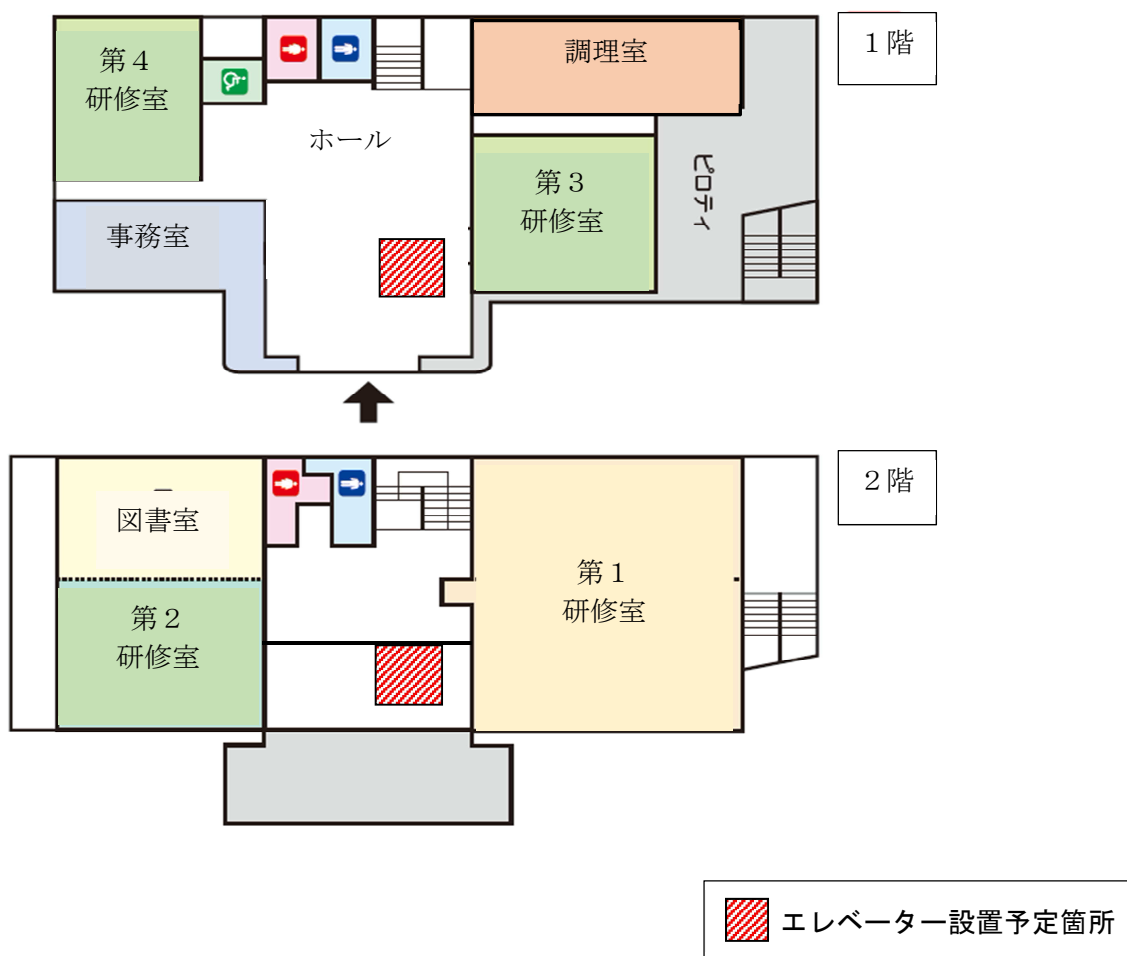
平面図
