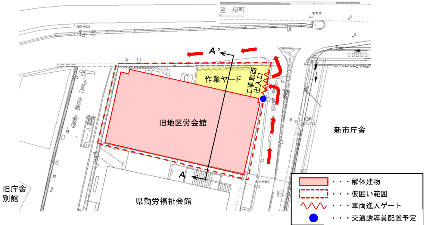
【 解体 平面図 】
