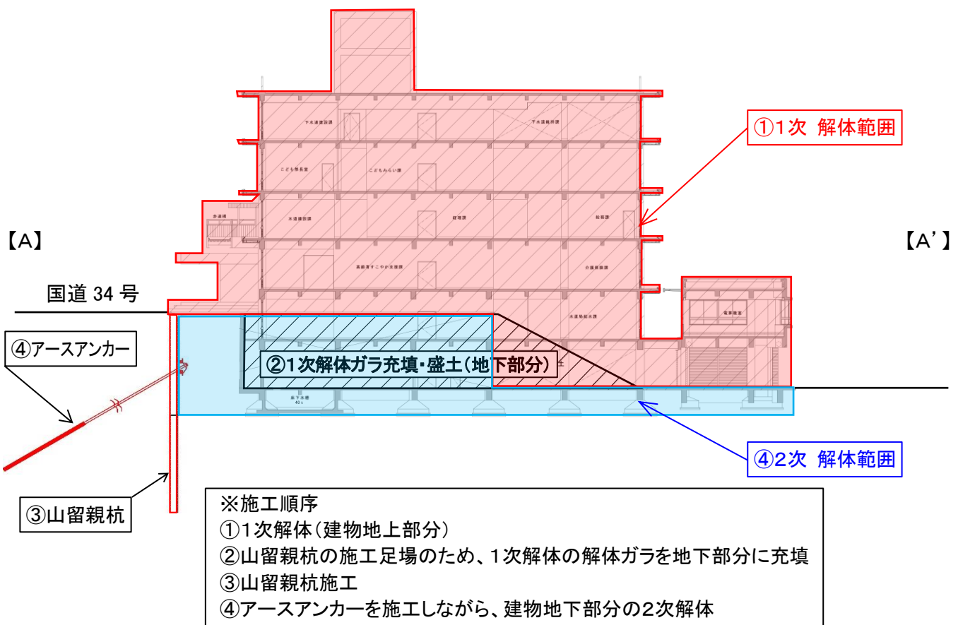
【 解体 施工順序図 】
