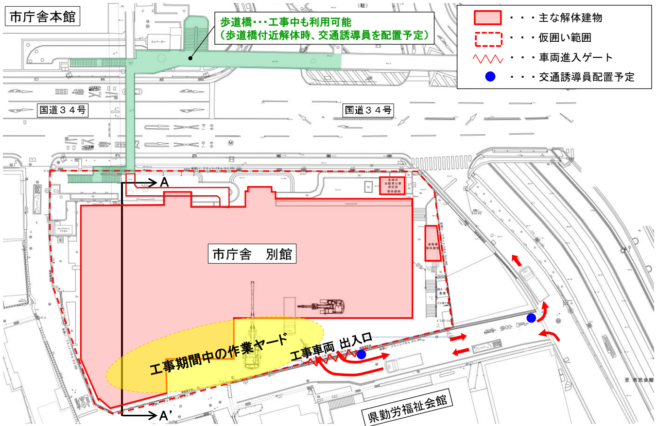
【 解体 平面図 】
