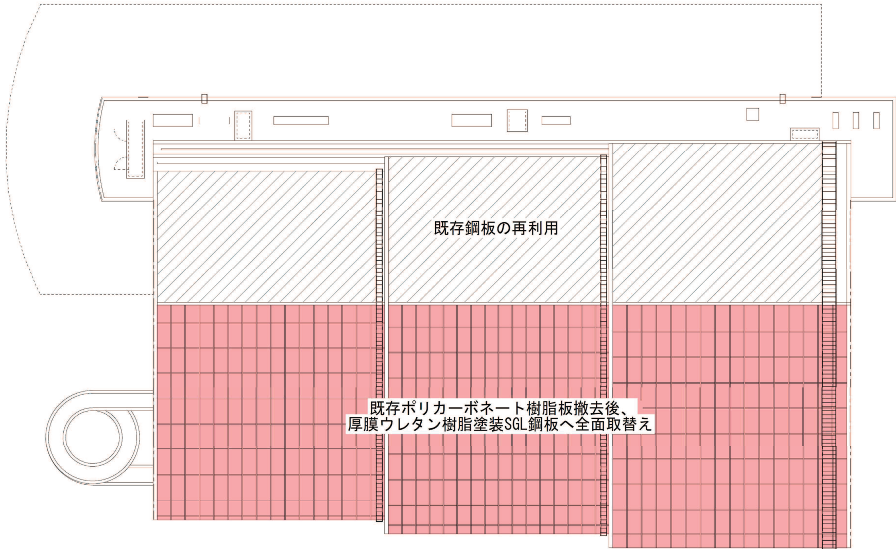
屋根伏図
