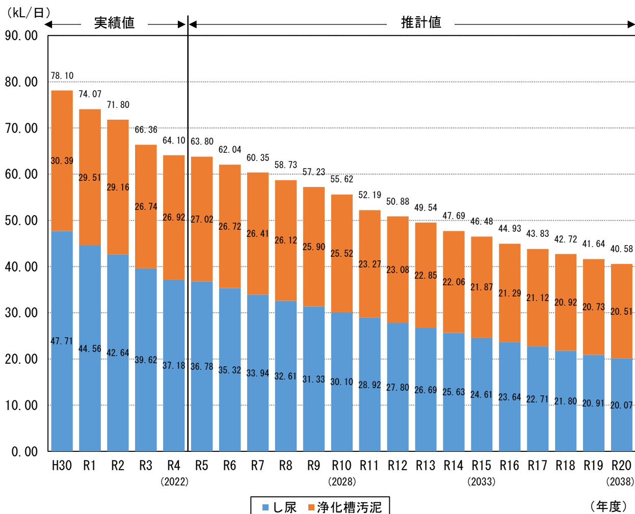
図 4-4 処理等発生量の推計結果（集落排水の統合計画を考慮）
