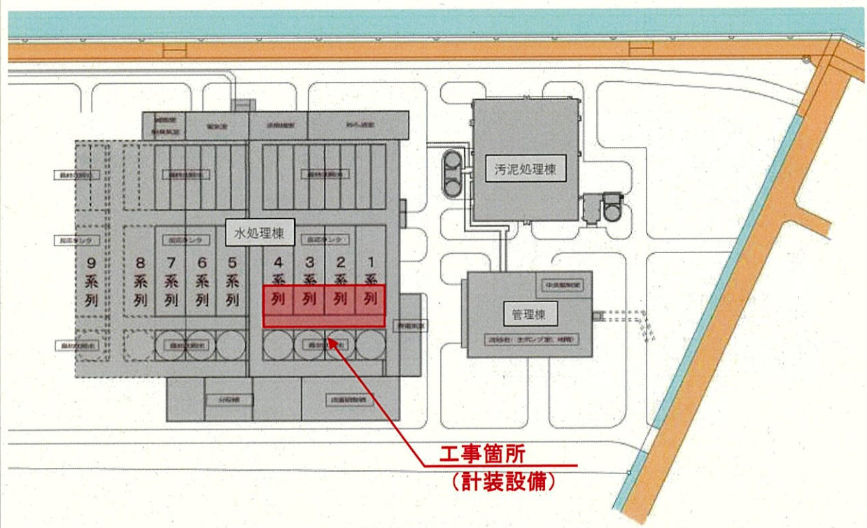
西下水処理場平面図
