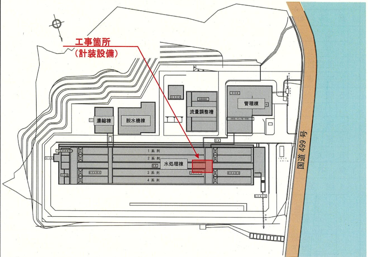
南下水処理場平面図
