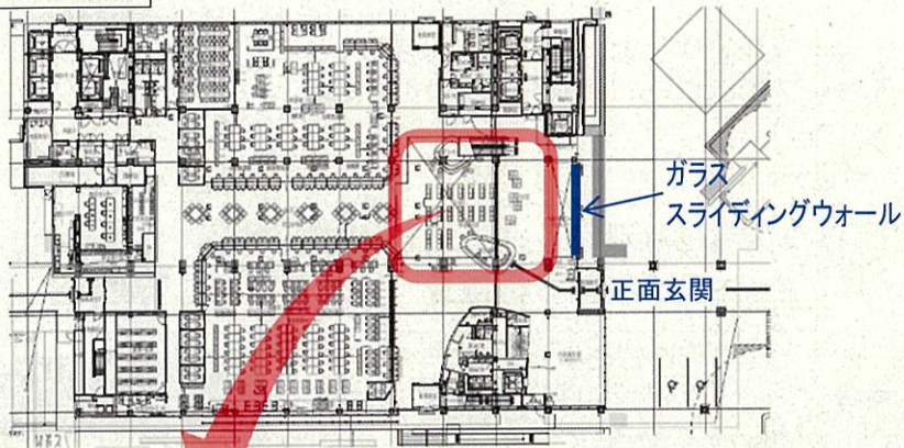
1階 平面図
