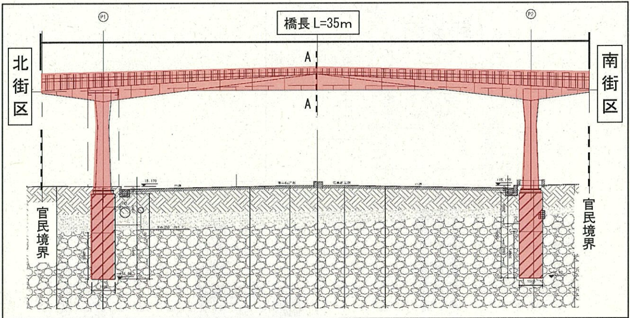
○立面図
