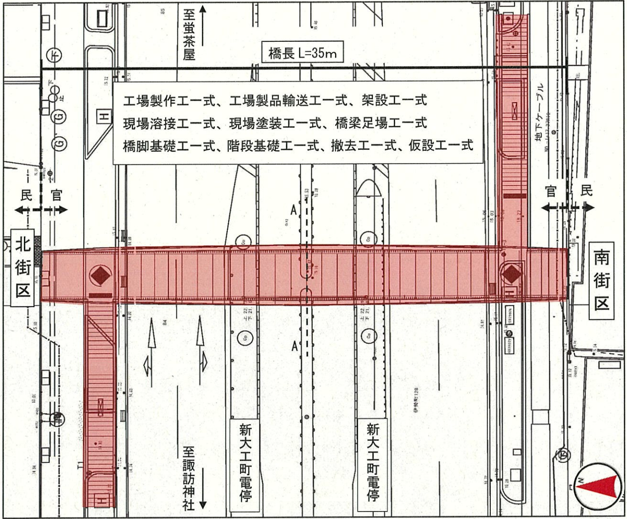
○平面図
