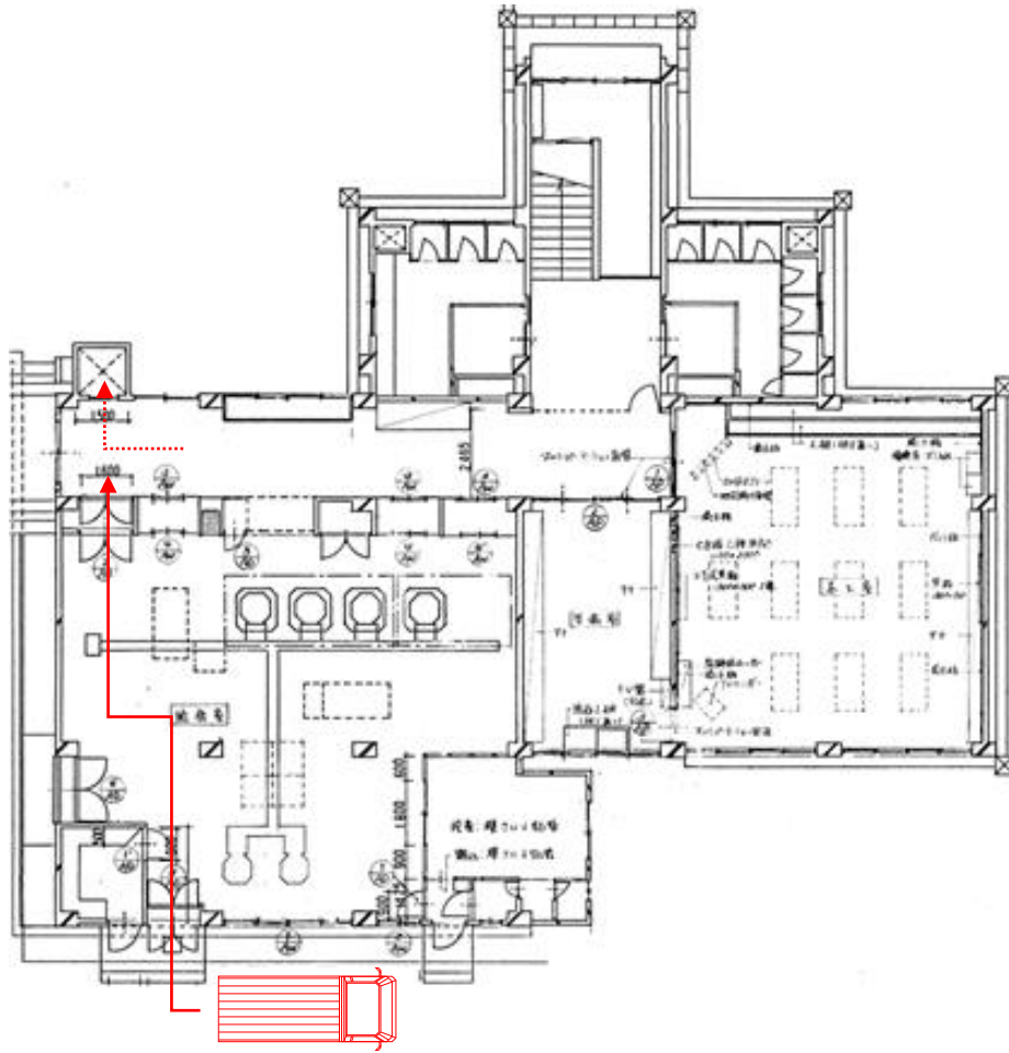
稲佐小学校 コンテナ配置図
