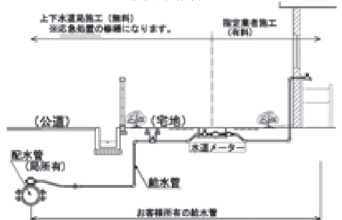
給水装置標準図
