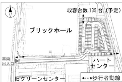
▲茂里町駐車場の整備イメージ図
