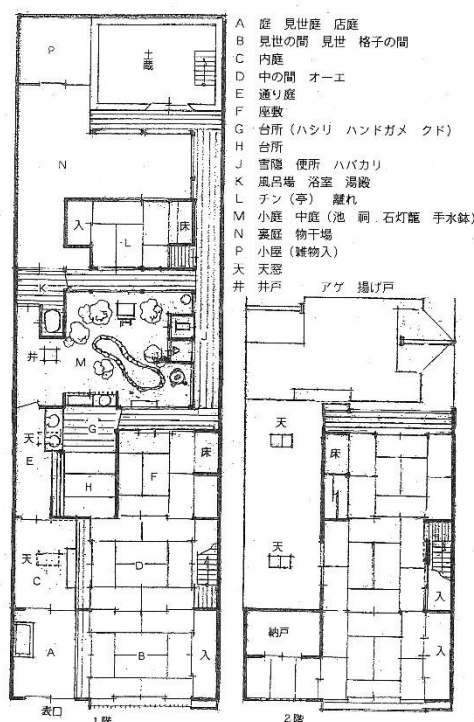
土蔵を有する町家の間取り図 （『長崎町人誌第6巻』より転載）
