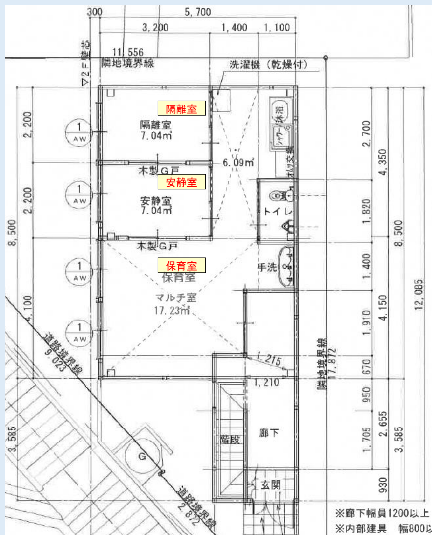
1 階 平 面 図
