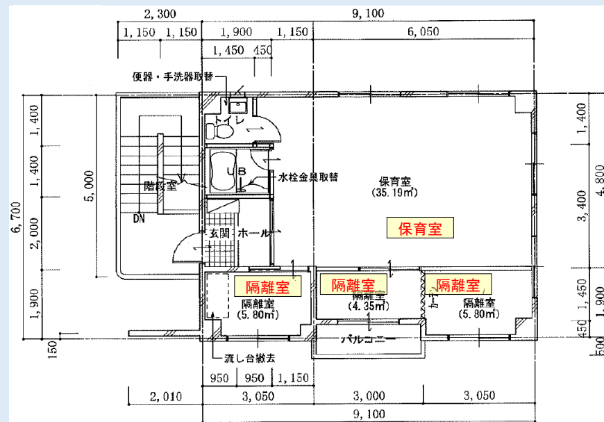
3 階 平 面 図
