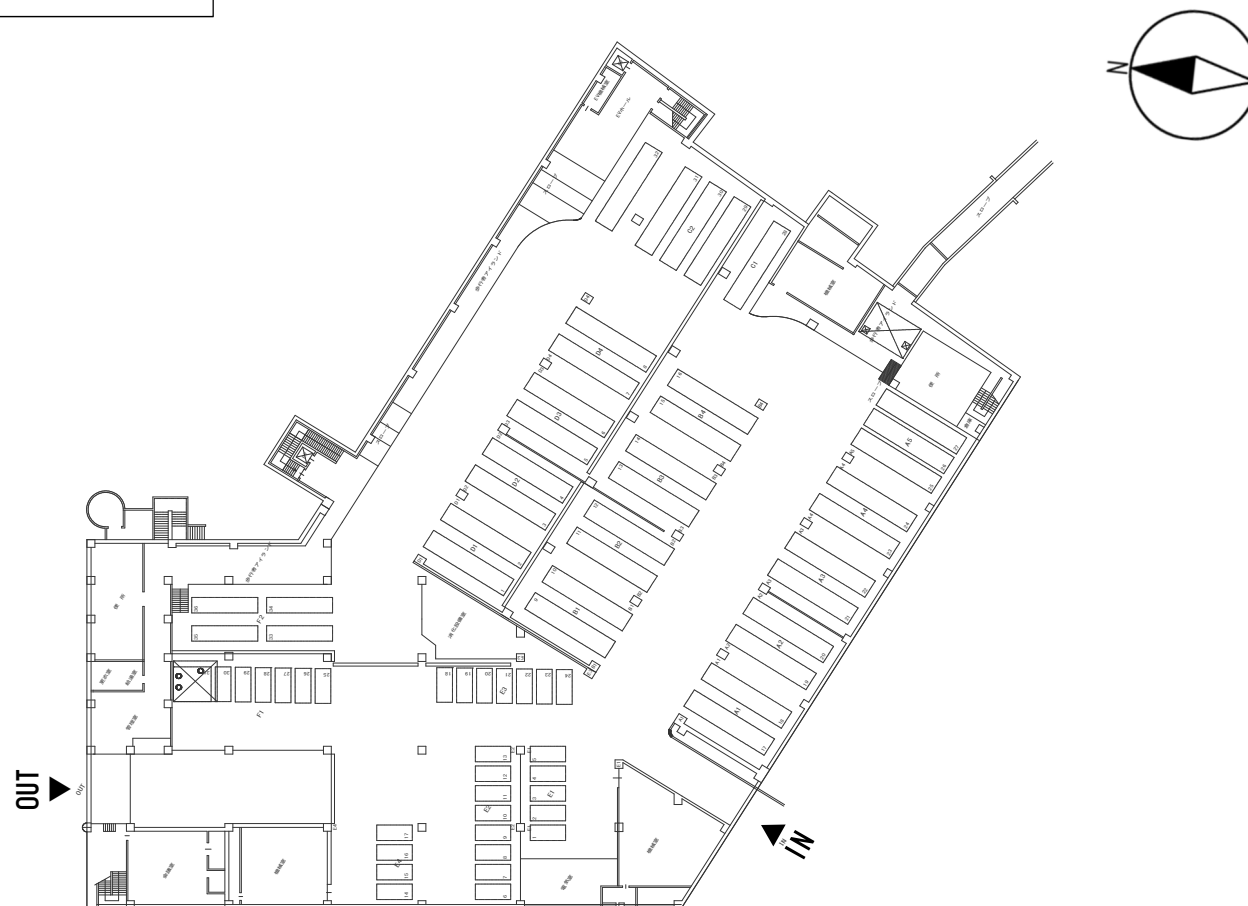
地下 1 階平面図
