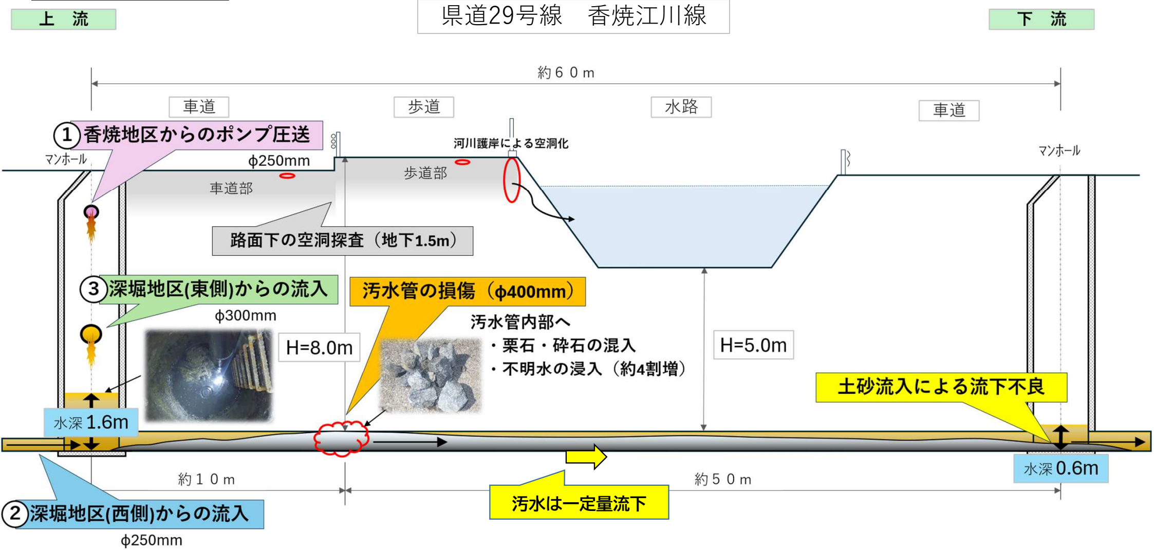
污水管損傷のイメージ
