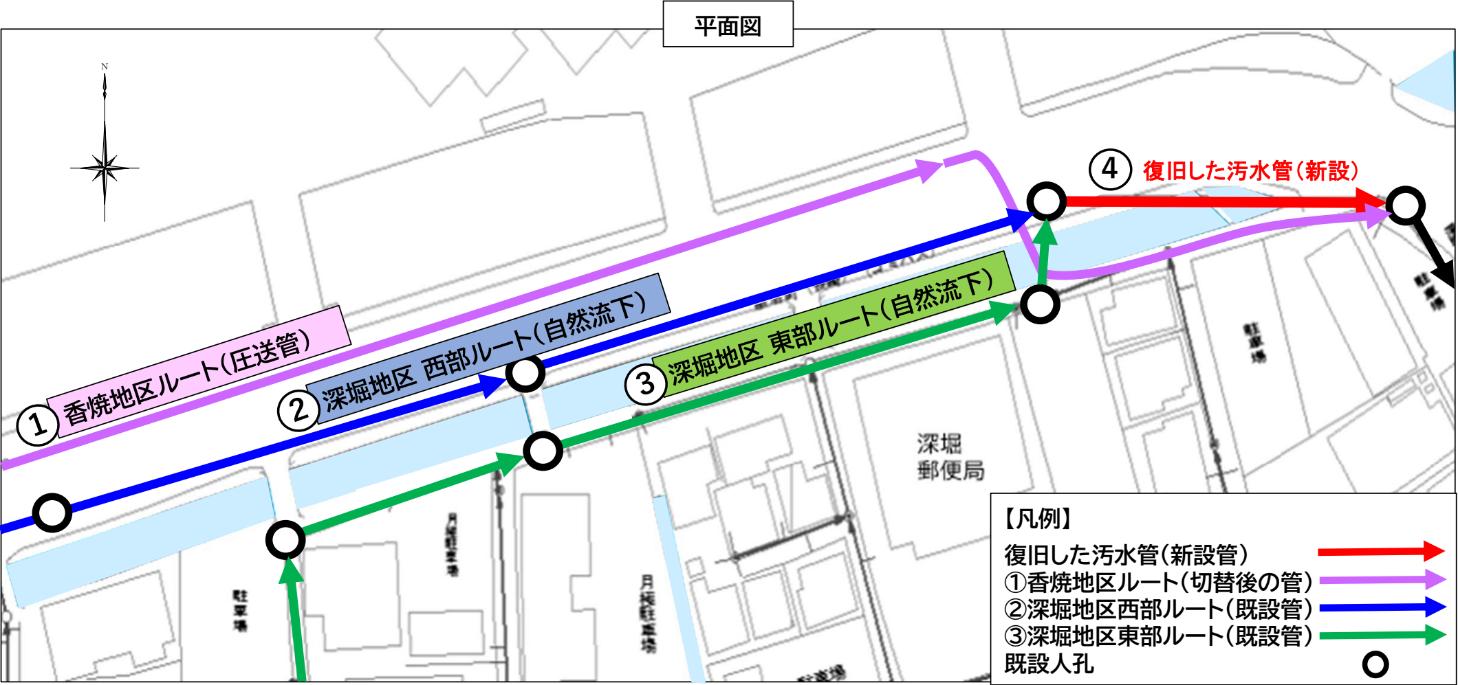
工事完成後の污水管
